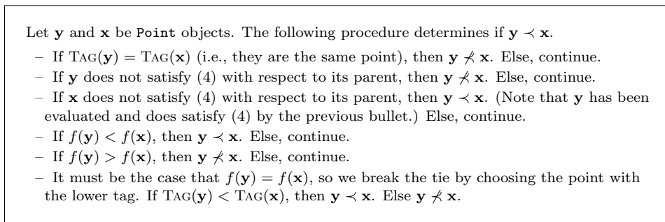
Fig. 2. Determining if \mathbf{y} \prec \mathbf{x} .
