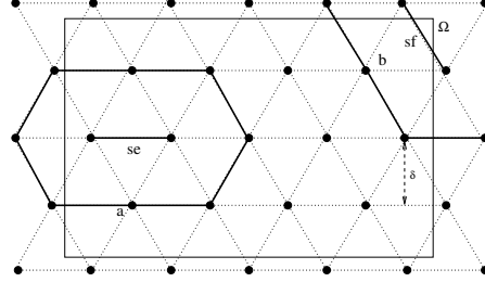
(d) Boundary superedge sets for superedges se and sf .
