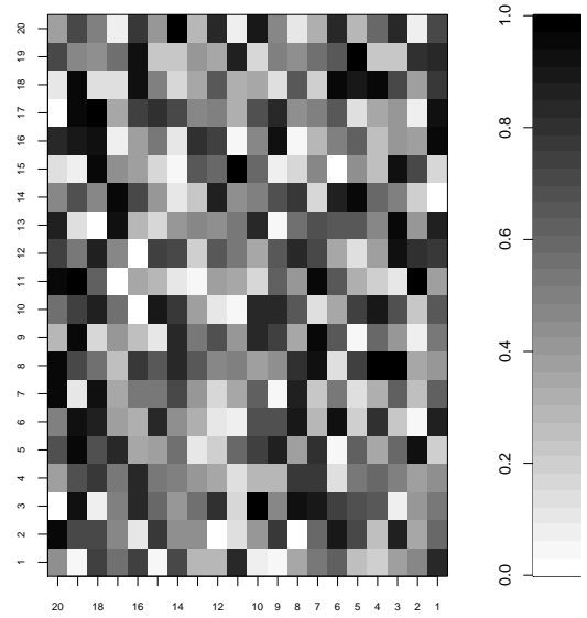
(d) A structure free transition matrix
